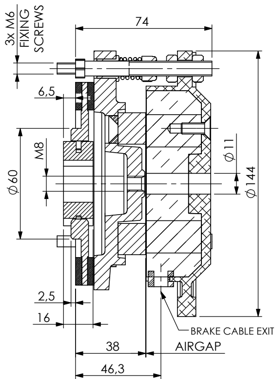
SEZIONE A-A SCALA 1 : 2
