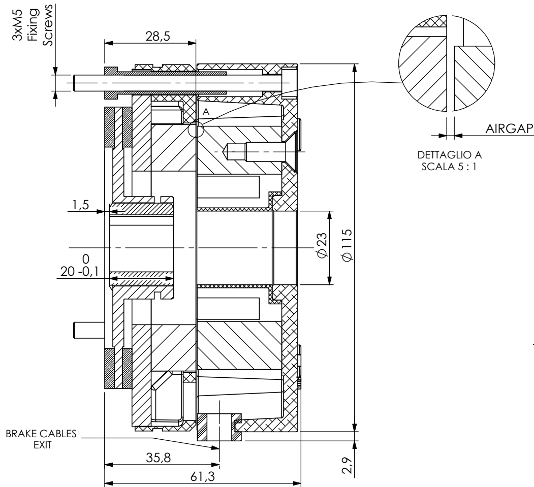
SEZIONE H-H
