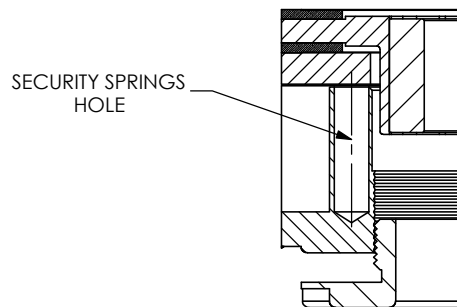
SEZIONE B-B
